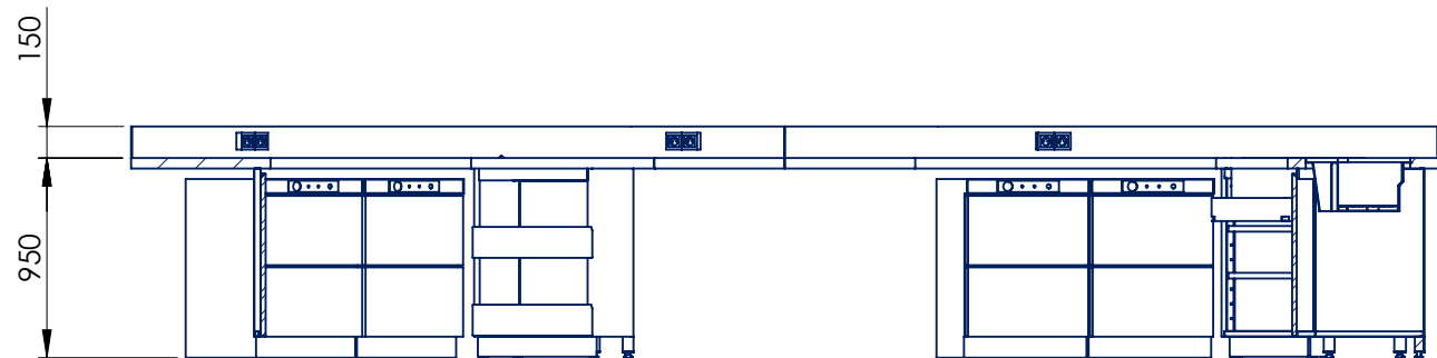
SECTION A-A
